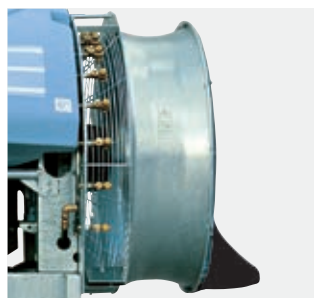
Protezione contro l'aspirazione di corpi estranei / Fan protection against leaves and soil remains / Protection pour empêcher l'aspiration des feuilles / Blätterschutz / Protección contra la aspiración de hojas
