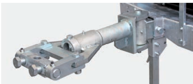
Timone sterzante con cuscinetti tipo Germania / Tracker drawbar with bearings "German type" / Attelage articulé monté sur roulement modèle Germania / Lenkdeichsel mit Lager Germania Modell / Tiro articulado con cojinetes tipo Alemania
