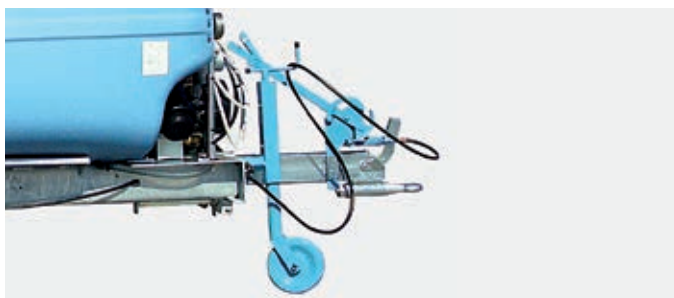
Ruotino appoggio / Tourning wheel / Support Béquille jockey / Stützrad / Rueda de apoyo
