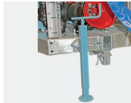
Piedino appoggio regolabile / Adjustable support / Béquille jockey sans roue / Verstellbarer Stützfuß / Apoyo adjustable
